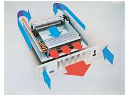
Effektive Kickspace trækker luft ind gennem sidetremmerne i frontpanelet. Ventilatoren fører luften gennem konvektoren, hvor den varmes op, og derefter tilbage i rummet gennem frontpanelets midterfelt.
